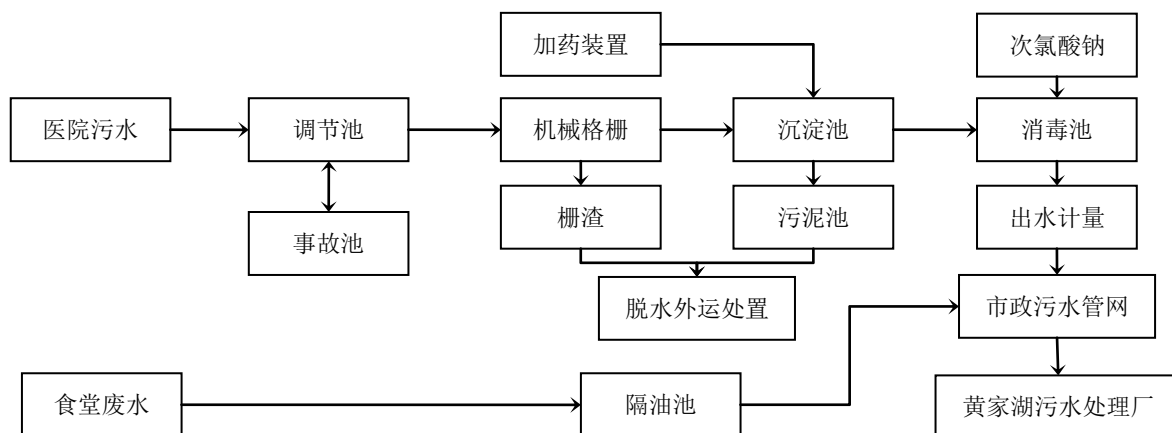
图 5-2-2 医院污水处理设施工艺流程图
